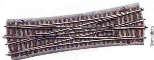
Стрелка двойной рельсовой крестовины
